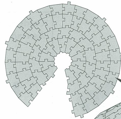
Spread out roof Chapiteau déployé
